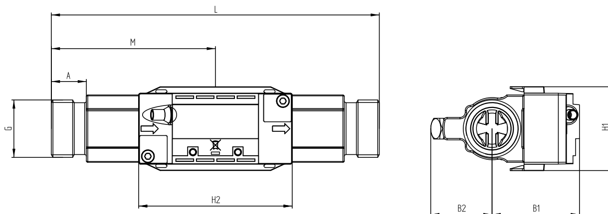
Mechanische Abmessungen der Elektronikeinheit
